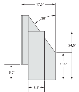
Seitenansicht
